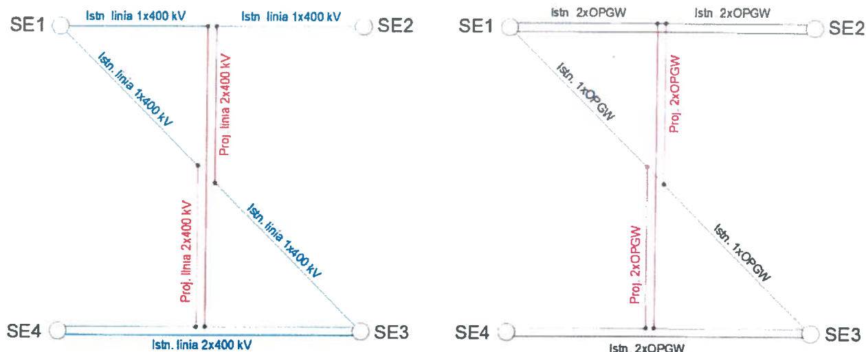
Rysunek 2. Stan planowany układu sieci 400 kV dla połączeń prądowych i odgromowych OPGW
