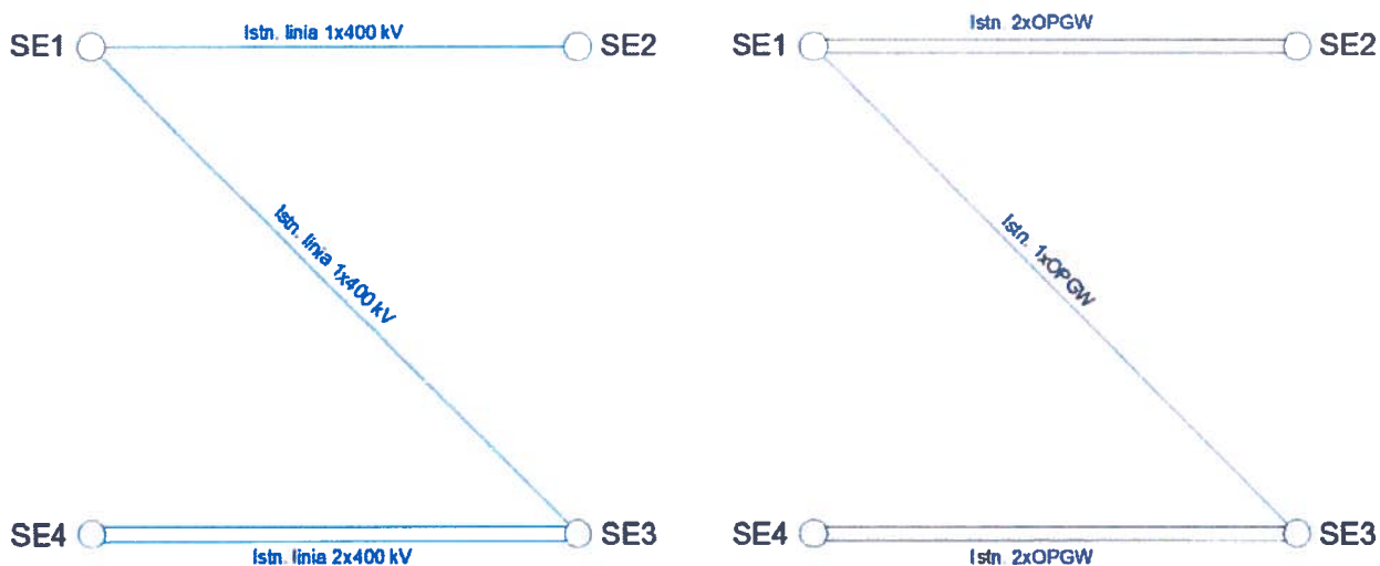
Rysunek 1. Stan istniejący układu sieci 400 kV dla połączeń prądowych i odgromowych OPGW
